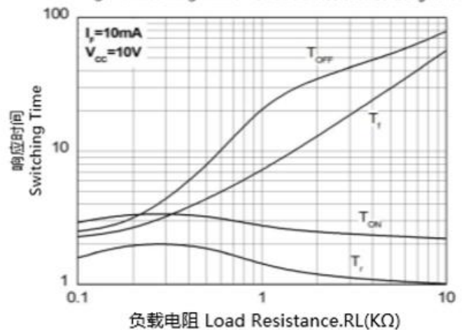
图6. 响应时间 vs 负载电阻曲线图 Fig.6 Switching Time vs. Load Resistance Diagram
